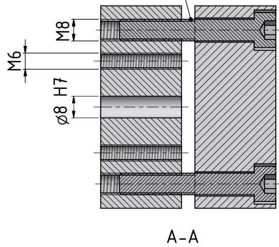
4x Klemmschraube clamping screw
